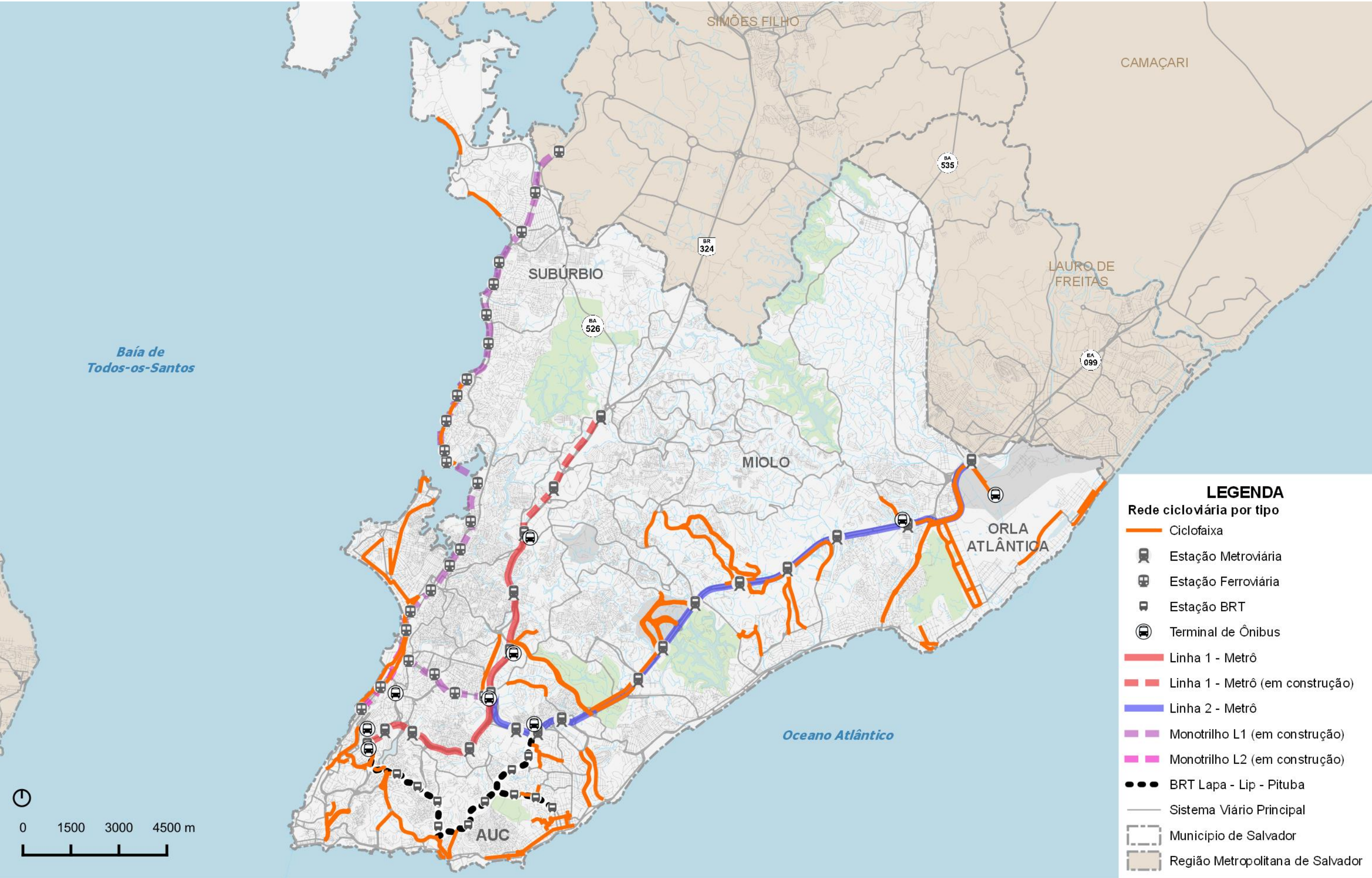
Figura 50 – Localização das ciclofaixas ao lado da calçadas Fonte: Elaboração Oficina Engenheiros Consultores Associados
