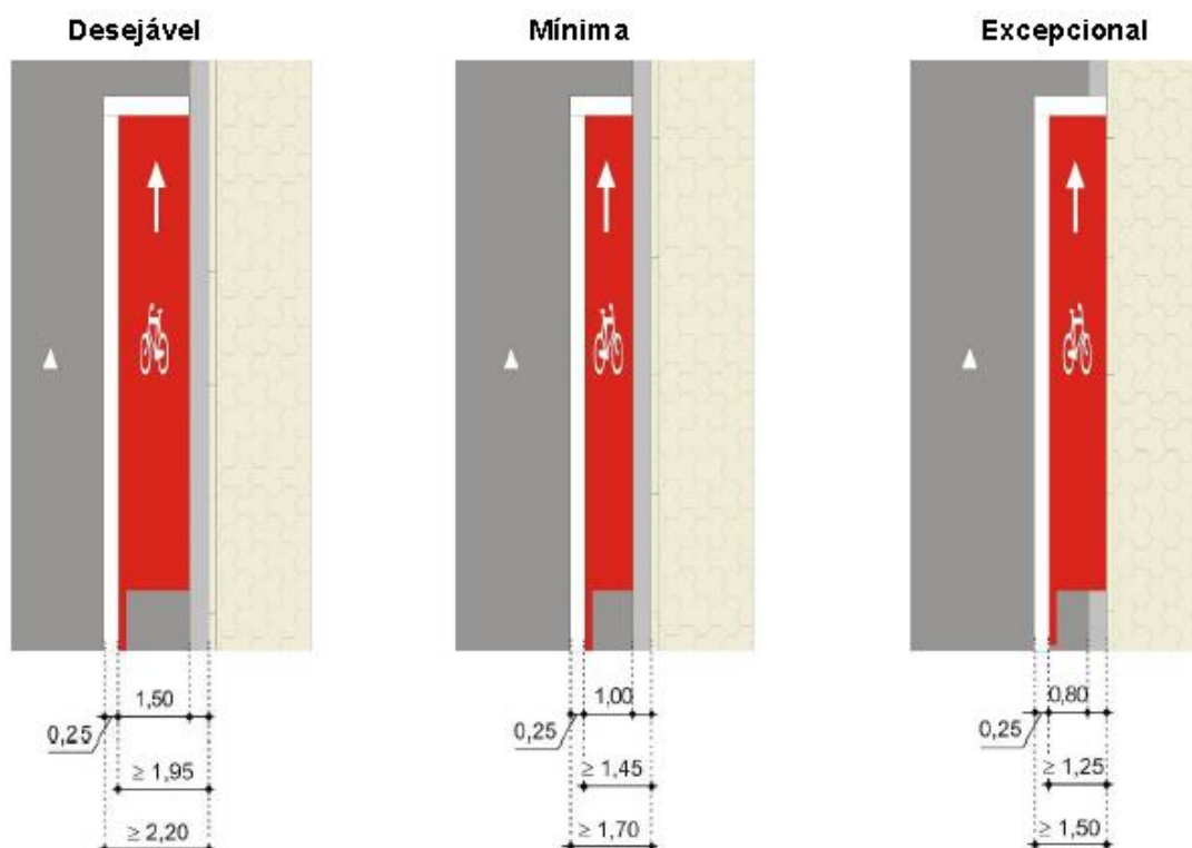
Figura 81 – Larguras para a solução de ciclovias ou ciclofaixas unidirecionais
