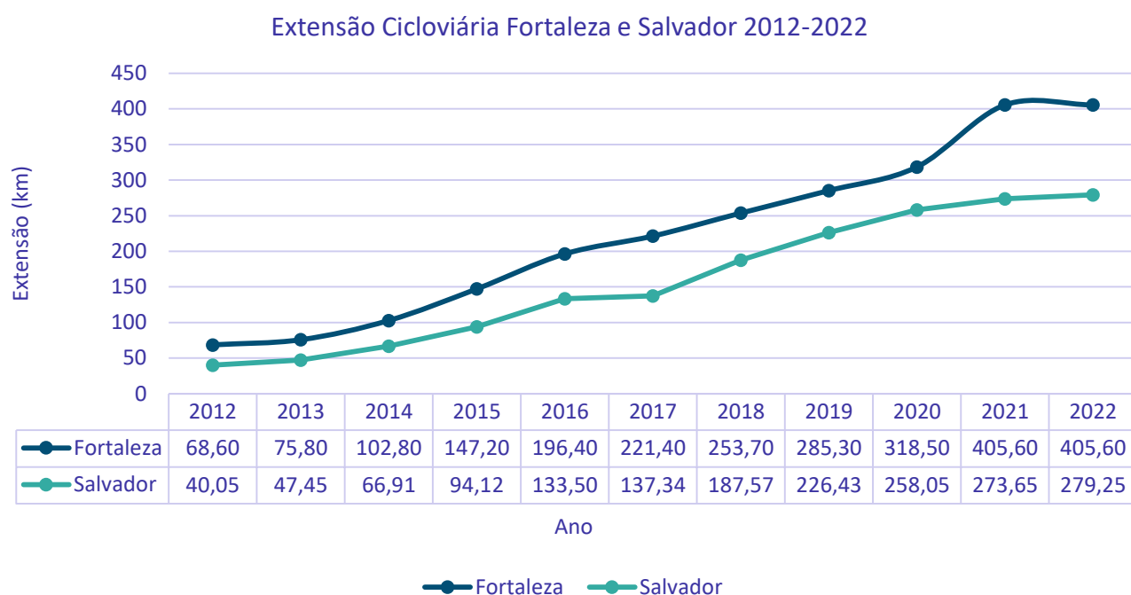
Figura 4 – Comparação da evolução da rede cicloviária de Salvador e de Fortaleza Fonte: Transalvador, maio/2022 e Plano de Acessibilidade de Fortaleza, 2021
