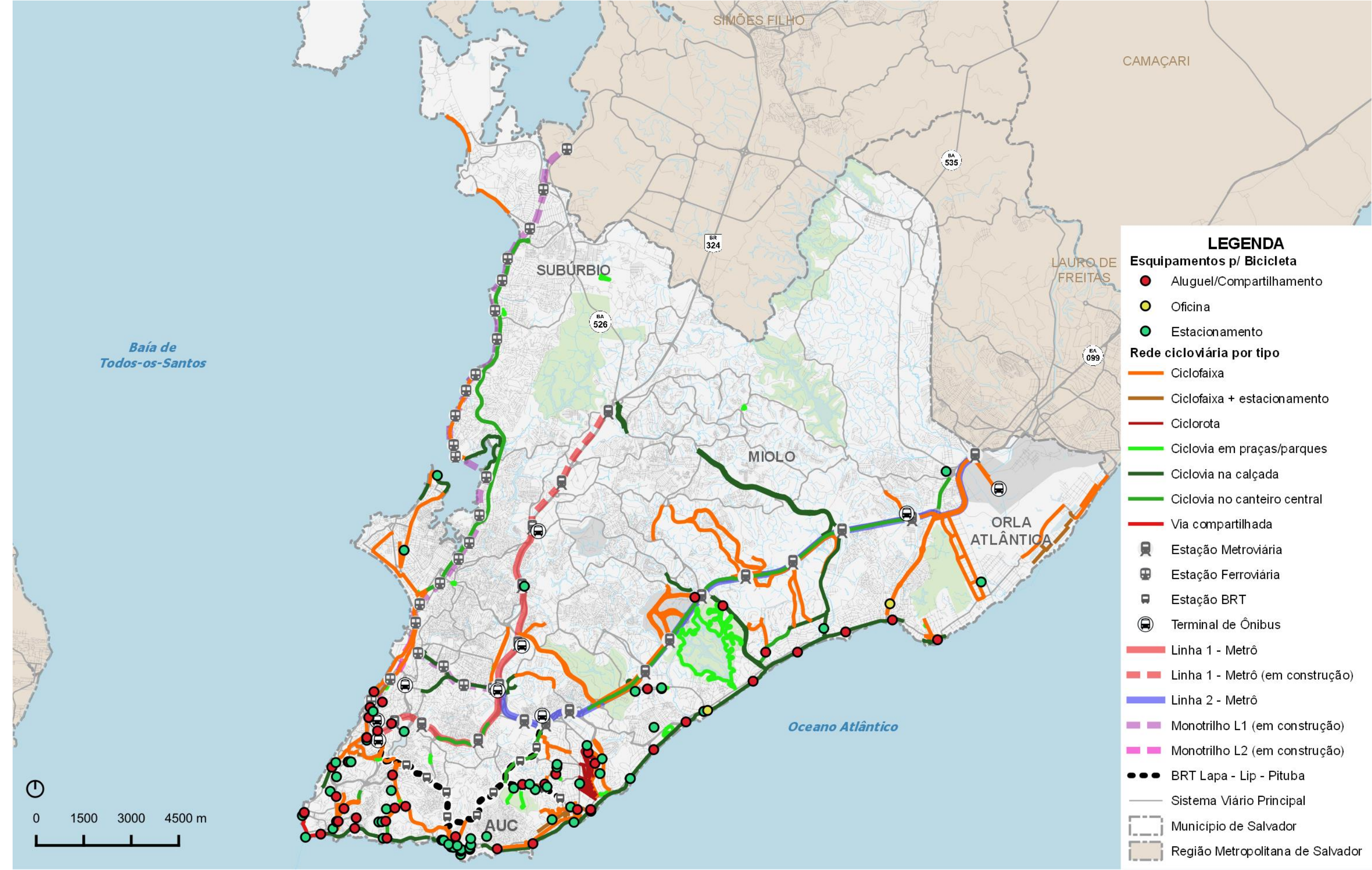
Figura 117 – Localização de equipamentos para bicicletas Fonte: Elaboração Oficina Engenheiros Consultores Associados
