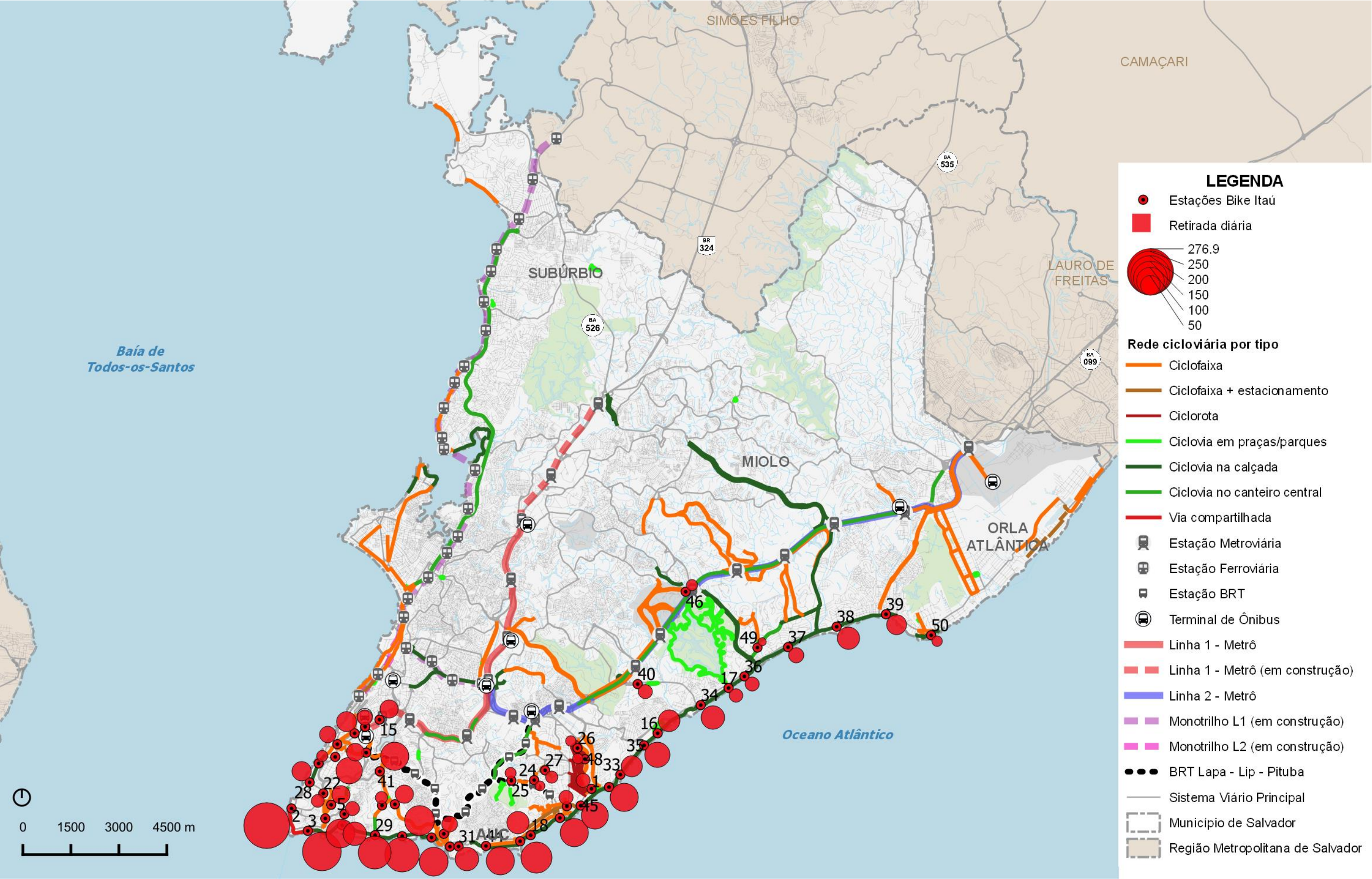
Figura 131 – Retiradas por estação em sua média diária Fonte: Elaboração Oficina Engenheiros Consultores Associados
