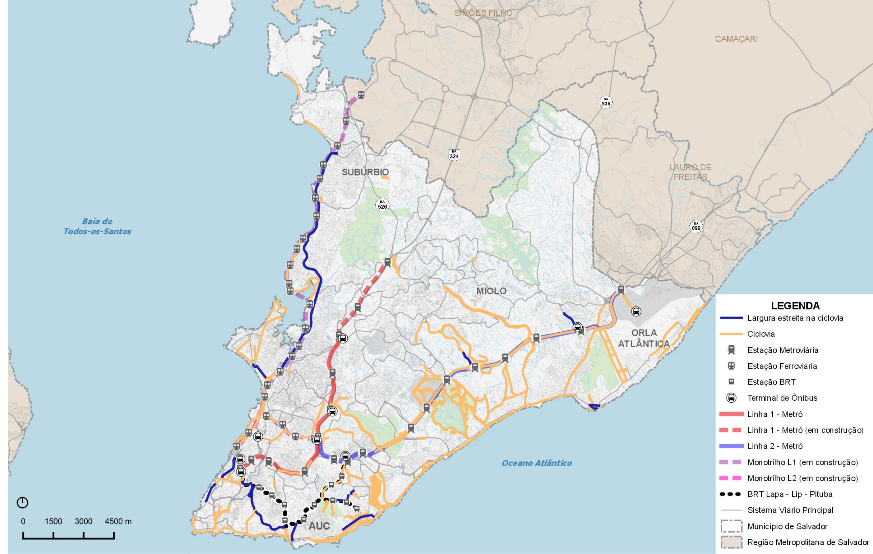
Figura 85 – Trechos com larguras inadequadas e necessidade de bidirecionalidade no tratamento cicloviário
