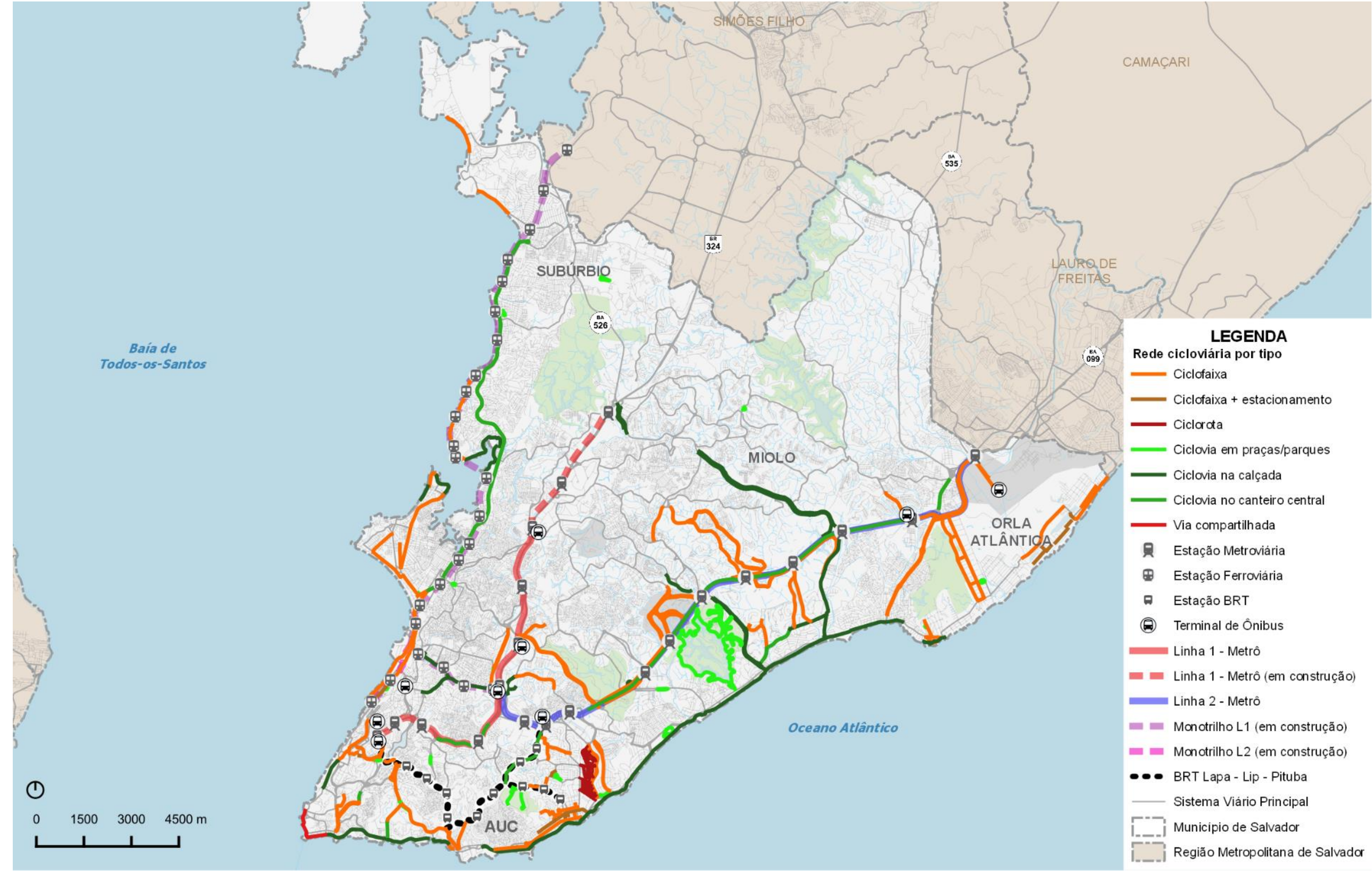
Figura 2 – Rede ciclovária atual em Salvador
