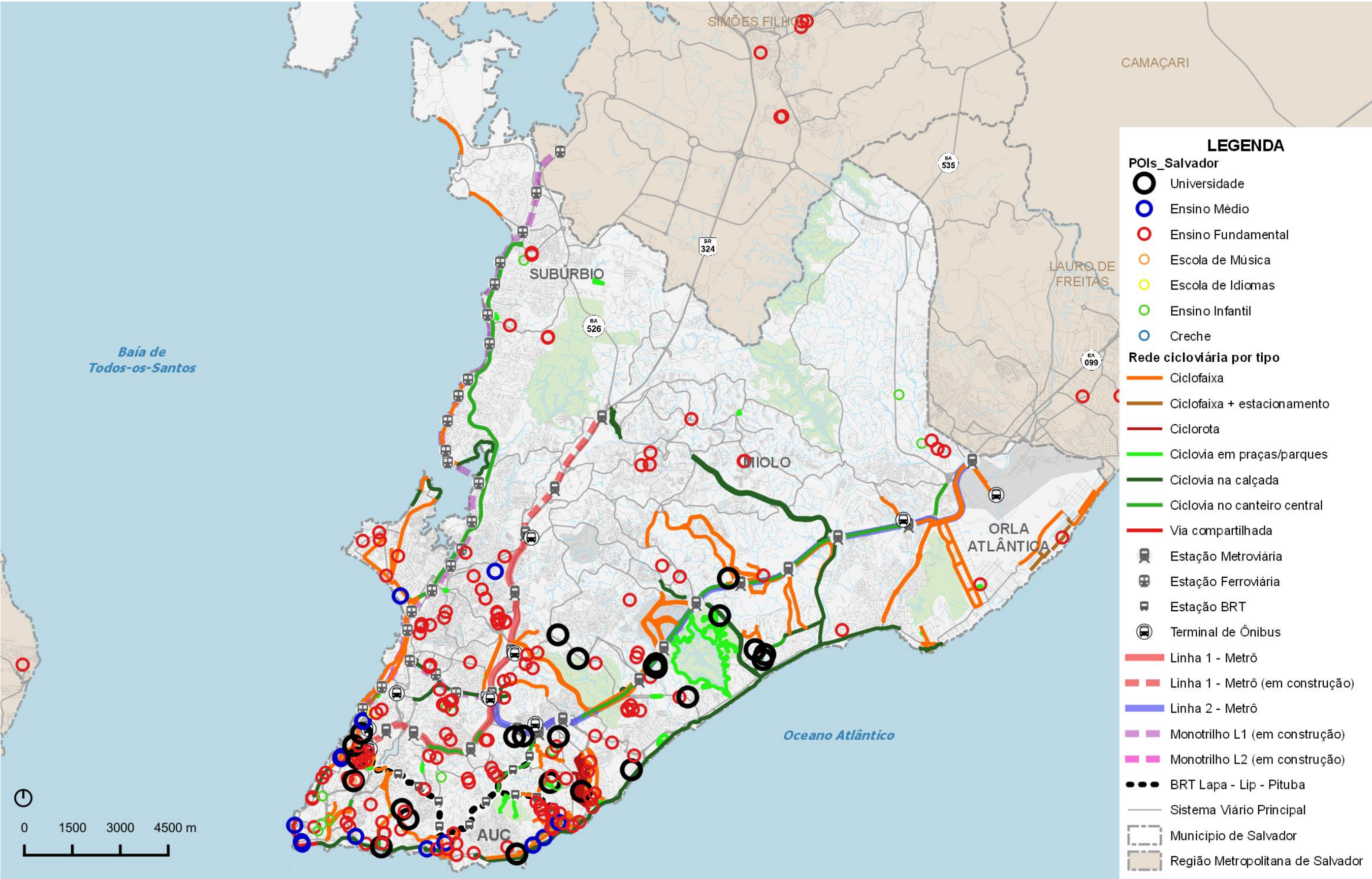
Figura 144 – Localização dos polos educacionais e atendimento pela rede ciclovitária Fonte: Elaboração Oficina Engenheiros Consultores Associados
