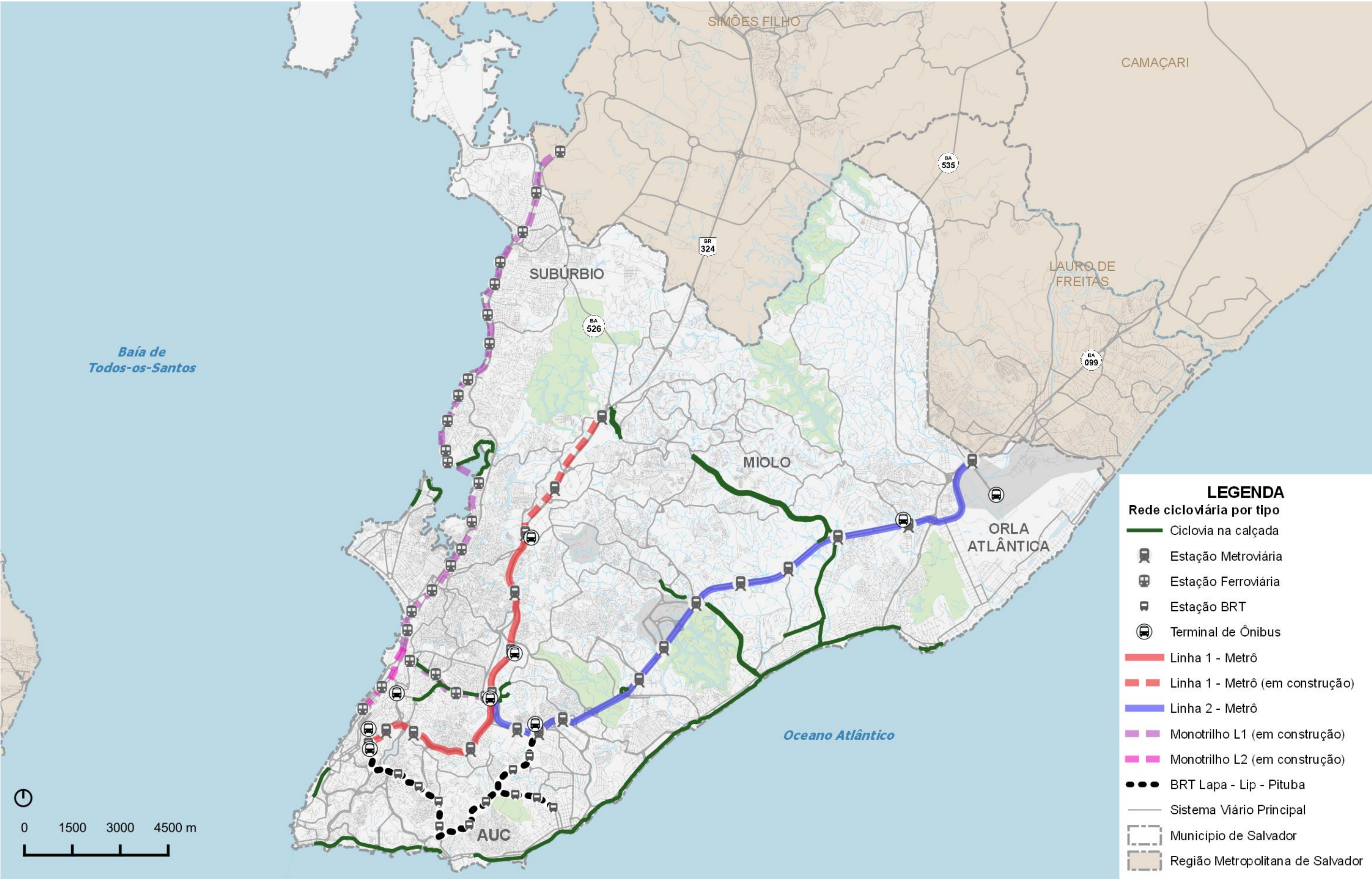
Figura 30 – Localização das ciclovias na calçada Fonte: Elaboração Oficina Engenheiros Consultores Associados
