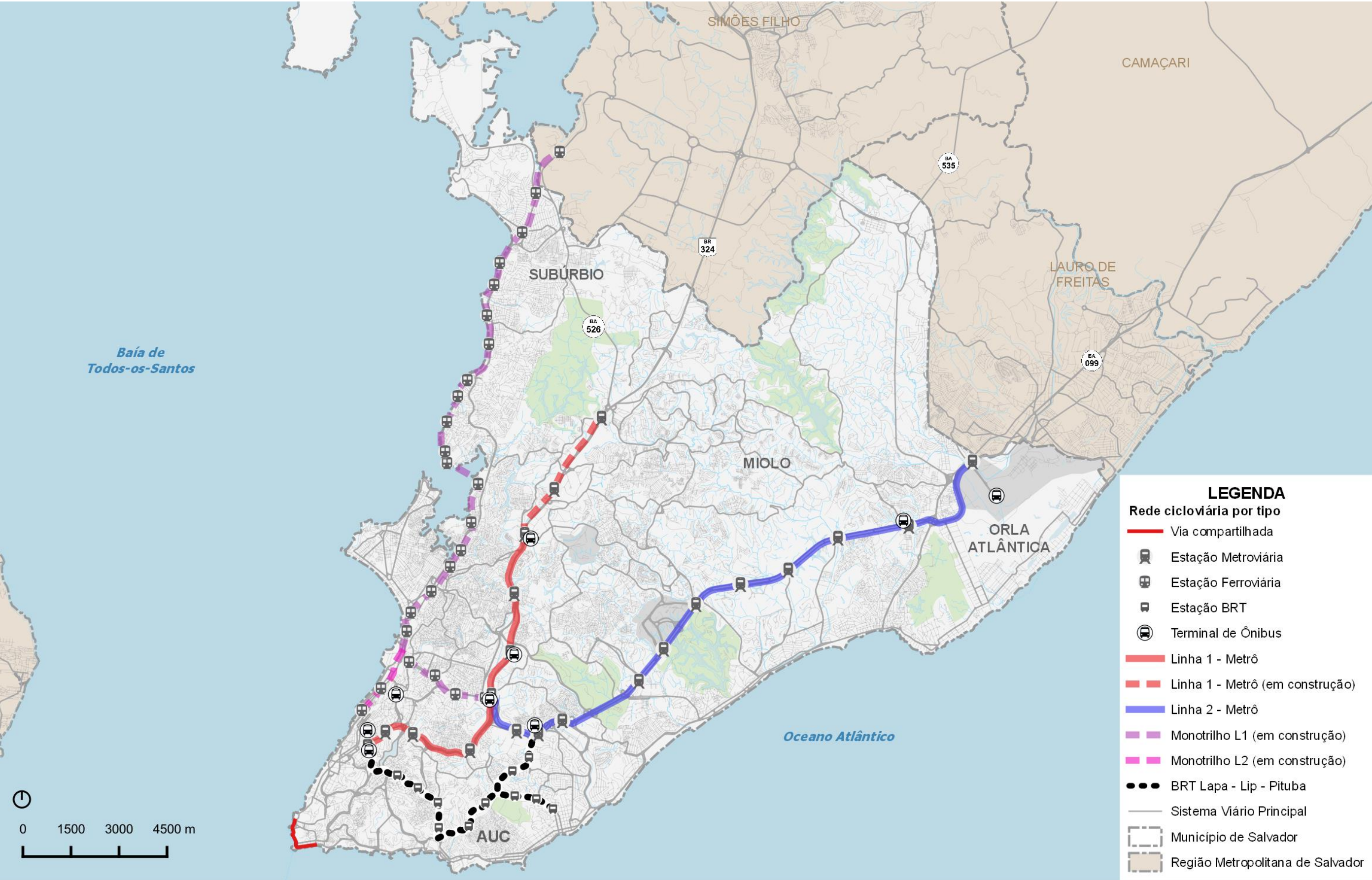
Figura 74 – Localização das vias compartilhadas Fonte: Elaboração Oficina Engenheiros Consultores Associados
