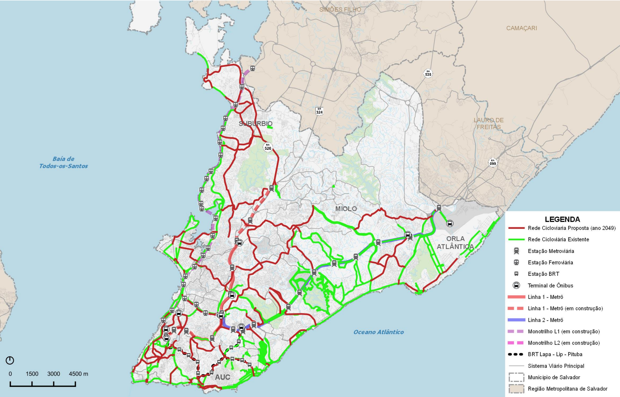
Figura 142 – Proposta de novos tramos cicloviários para o ano horizonte de 2049 do Planmob Salvador Fonte: Planmob Salvador, 2017
