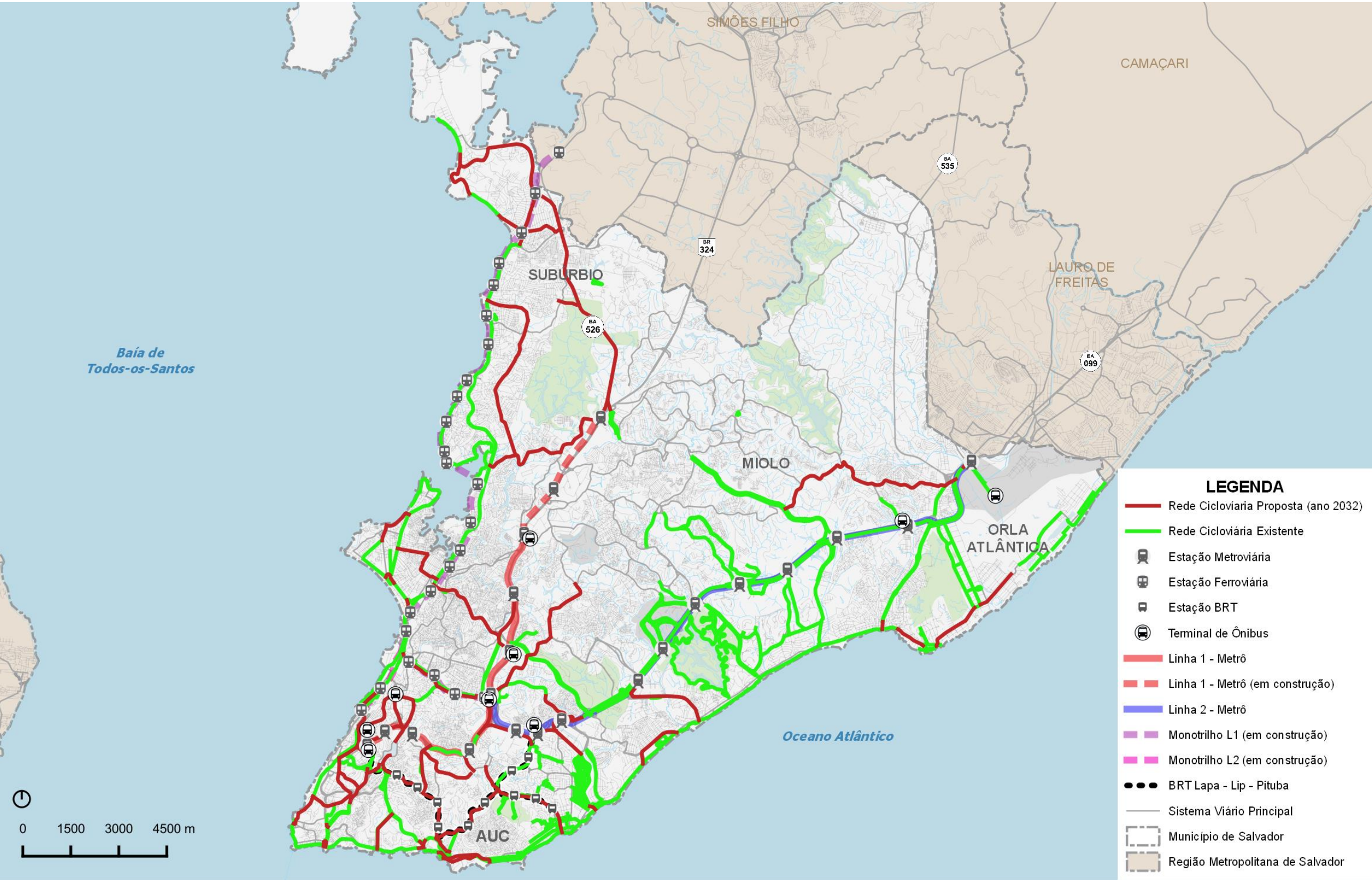
Figura 141 – Proposta de novos tramos cicloviários para o ano horizonte de 2032 do Planmob Salvador Fonte: Planmob Salvador, 2017
