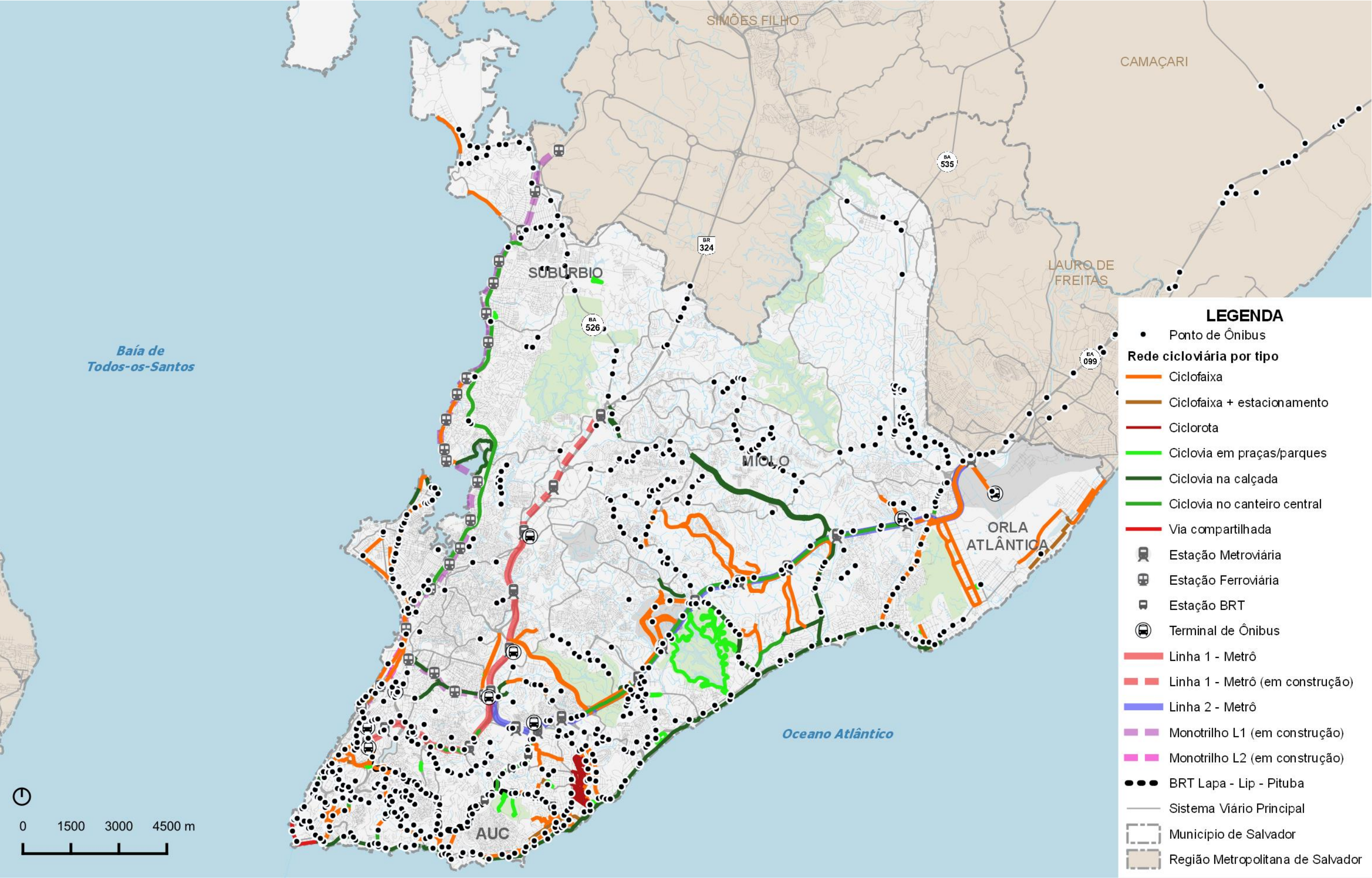
Figura 136 –Localização dos pontos de parada dos ônibus em Salvador e a rede cicloviária existente Fonte: Elaboração Oficina Engenheiros Consultores Associados
